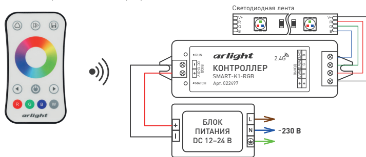
Рисунок 1. Схема подключения панели SMART-RGB-SET-RING
