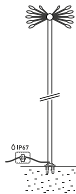
Рис. 3. Установка светильника на твердую поверхность
