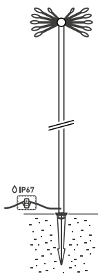
Рис. 2. Установка светильника в грунт
