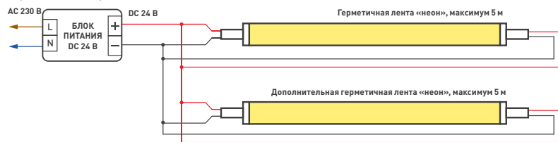
Схема 1. Подключение нескольких герметичных лент «неон»
